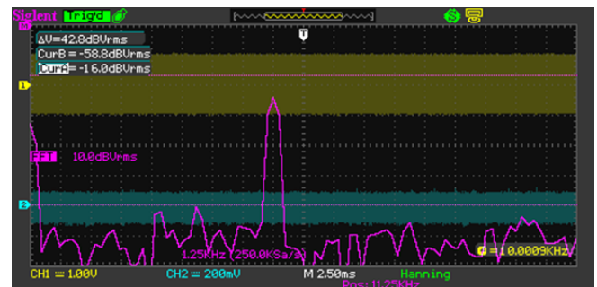
Fig. 11. FFT analysis
