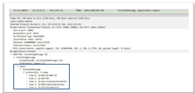
Fig. 15. Initial UE message
